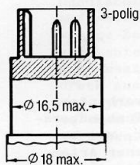
Stecker für Mikrofone nach DIN 41524
