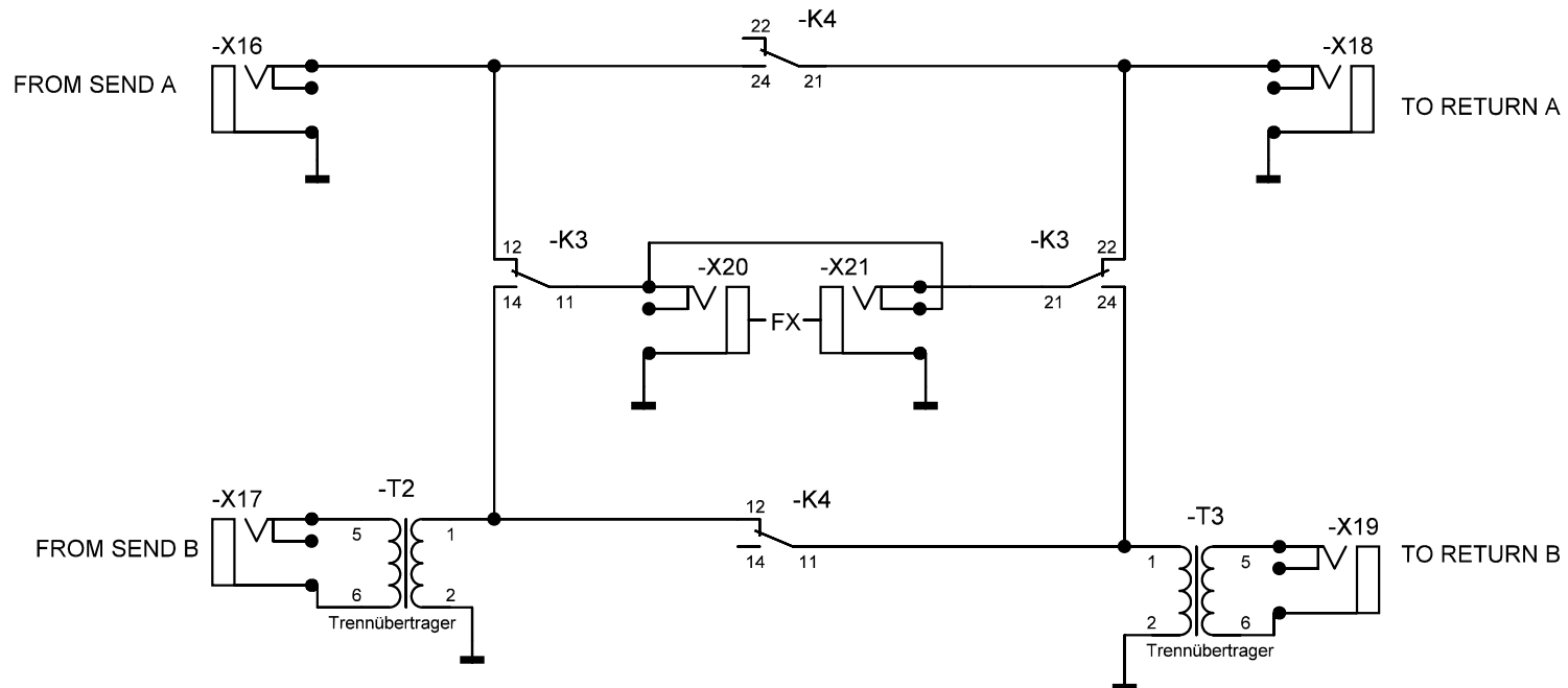
A/B/Y-Box - Umschleifen der Loop-Effekte Für 1:1-Übertrager 10 kOhm
