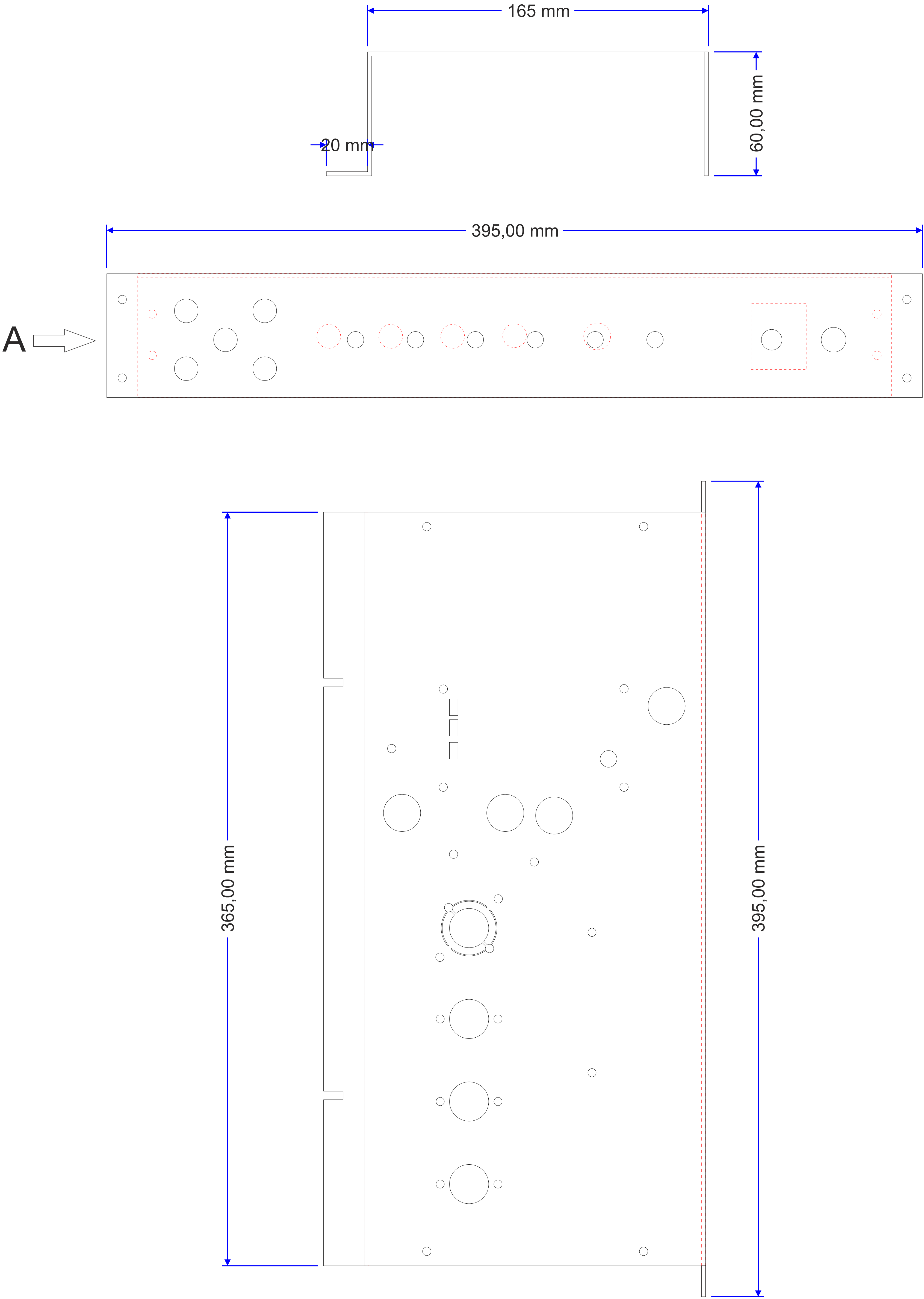
Seitenansicht A
